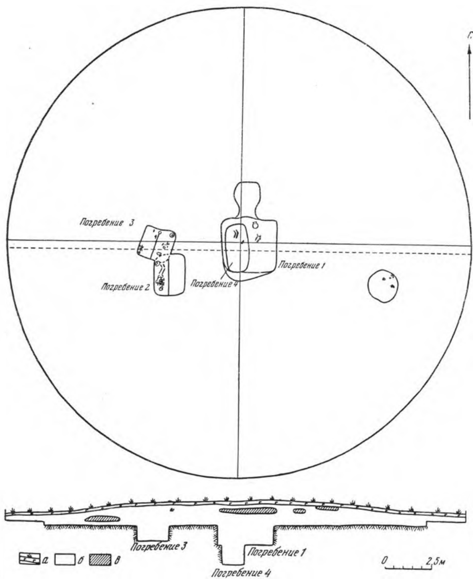
Рис. 13. План и профиль по линии запад-восток кургана 2 «Близнецы»:
